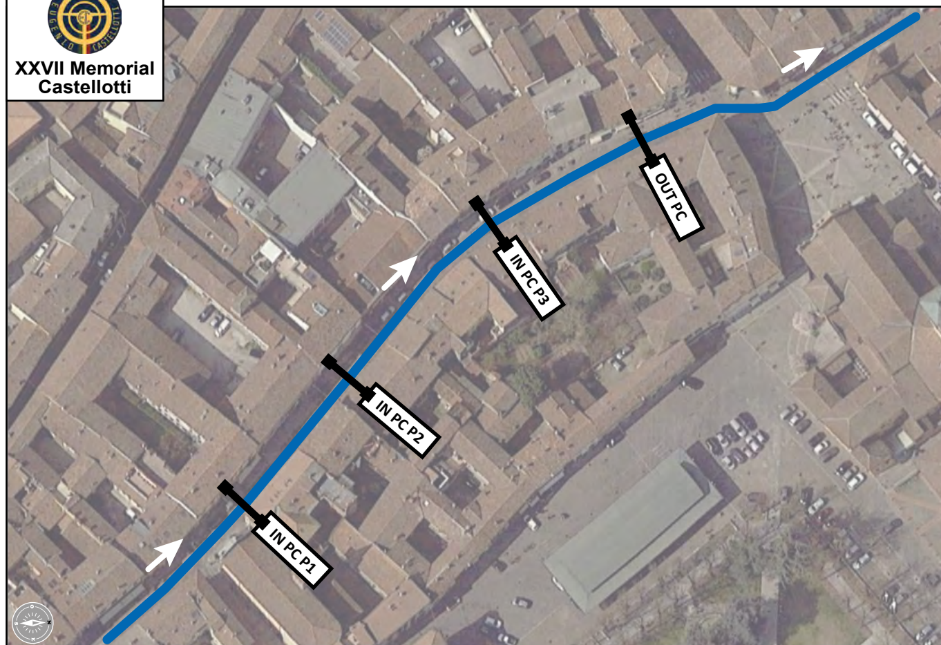
Planimetria 10 - Prove dalla P1 alla P3 - Power Stage Via Roma
