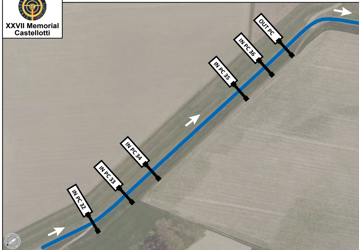
Planimetria 05 - Prove dalla 32 alla 36 - Lungopo
